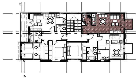
HORIZONTALNA DISPOZICIJA
